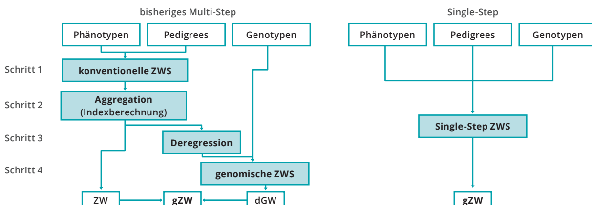
Abb. 1. Vergleich vom aktuellen Multi-Step-Verfahren mit der neuen Single-Step-Methode.
